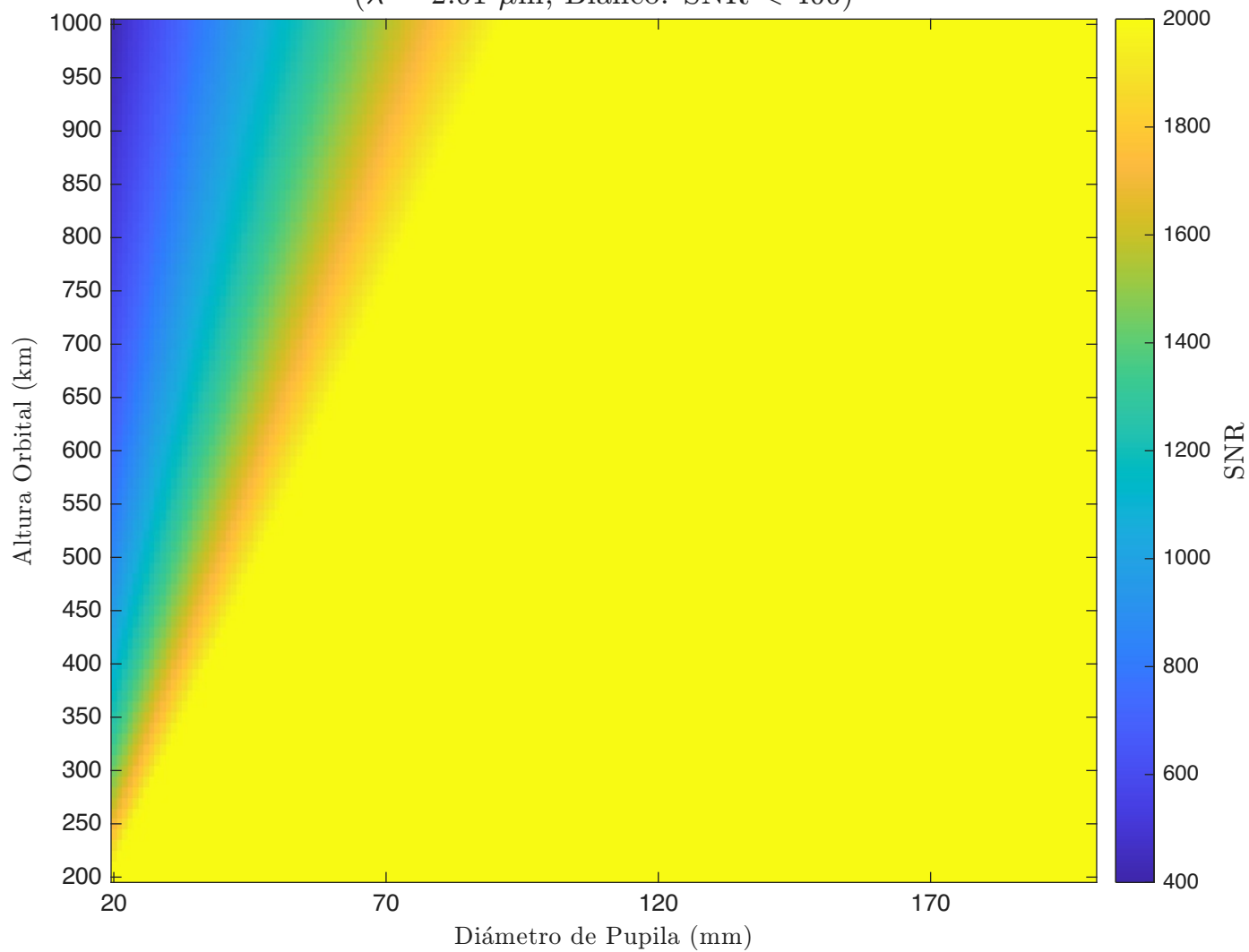
SNR - Cassegrain - Detector 1 ( \lambda = 2.01 \mu\text{m} , Blanco: SNR < 400)
